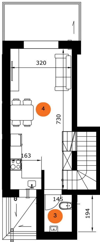
1 PIĘTRO
